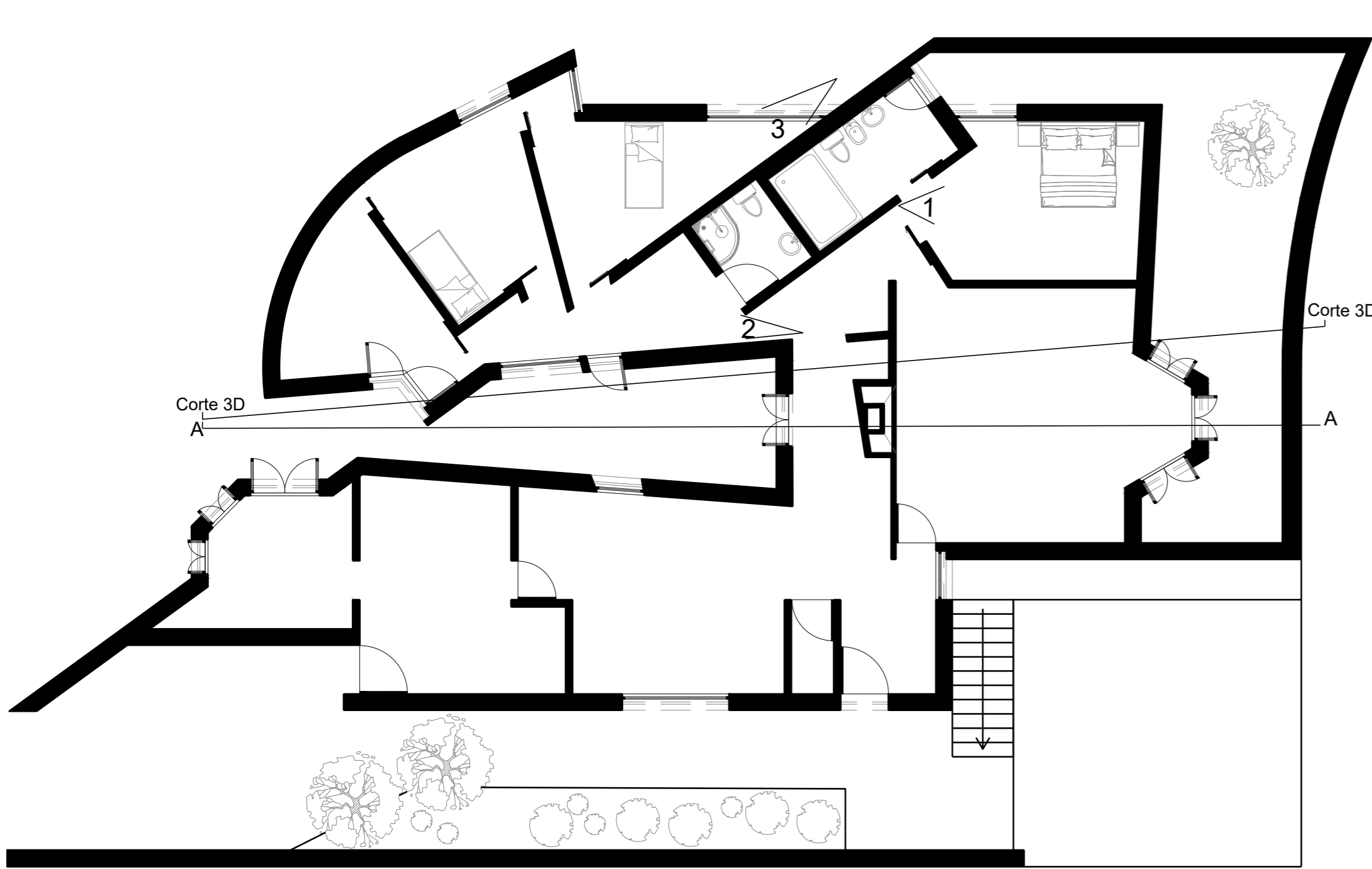
Planta esc.1/100
